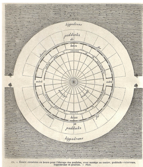
Plan d'une écurie circulaire en boxes
