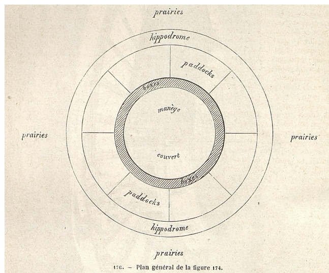
Plan d'une écurie circulaire
