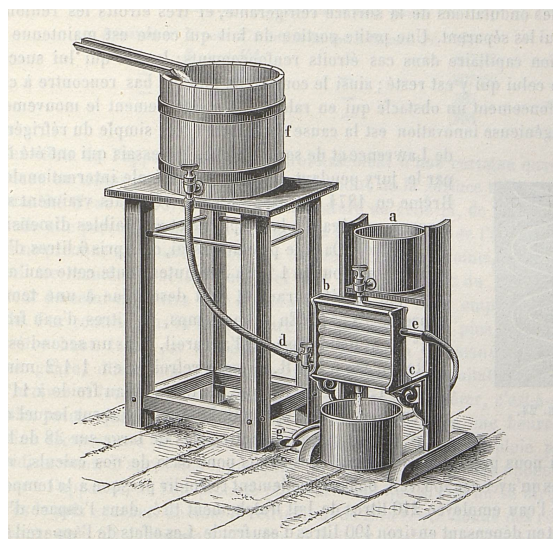
Réfrigérant de Lawrence
