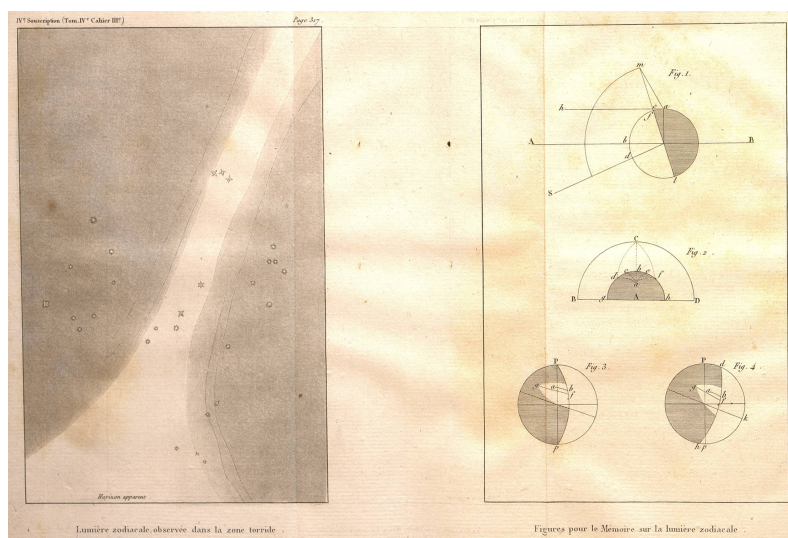
Lumière zodiacale observée dans la zone torride / Figures pour le Mémoire sur la lumière zodiacale
