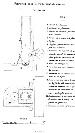
Fourneau pour le traitement du minerai de cuivre (fig. V)
